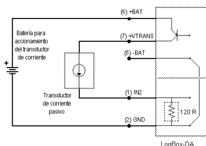
Figura 13 – Ejemplo de utilización del accionamiento externo
