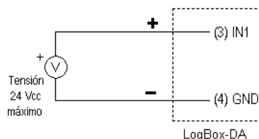
Figura 10 – Entrada tipo Pulso de Tensión y Contacto Seco para el canal 1
