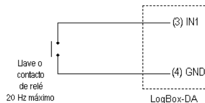
Figura 10 – Entrada tipo Pulso de Tensión y Contacto Seco para el canal 1
