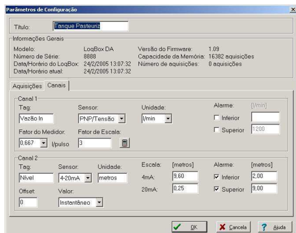
Figura 07 – Parâmetros de configuração de los canales de entrada
