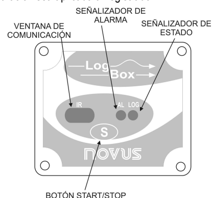
Figura 02 – Señalizadores y ventana de comunicación IR
