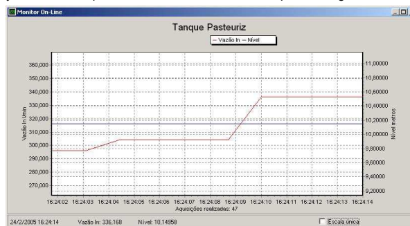
Figura 17 – Gráfico de monitorización on-line
