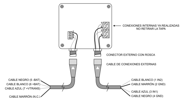
Figura 09 – Versión IP67, conectores externos
