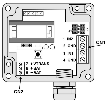
Figura 08 – Versión IP65, vista interna de las conexiones
