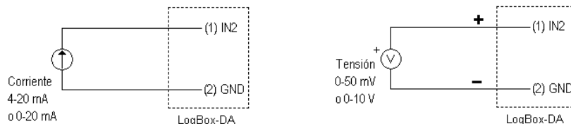
Figura 12 – Entradas de corriente y de tensión para el canal 2
