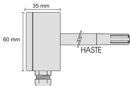
Fig. 07 - Dimensiones del modelo RHT/DM.
