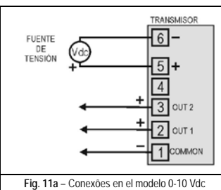
Fig. 11a - Conexões en el modelo 0-10 Vdc
