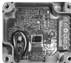
Fig. 09 - Localización de los Jumper J4 y J5 en el interior del transmisor
