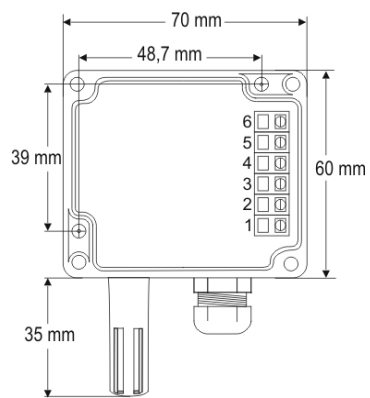
Fig. 08 - Agujeros de fijación y medidas do modelo RHT / WM.
